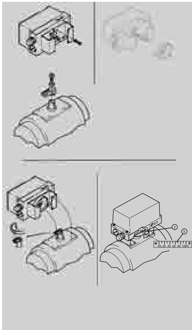
SITRANS VP100 在角行程执行机构上的安装
