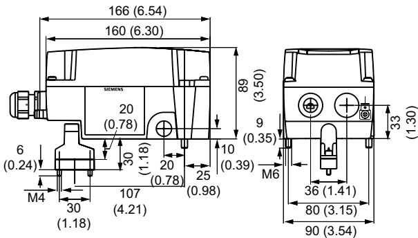
直行程执行机构，尺寸单位：mm
