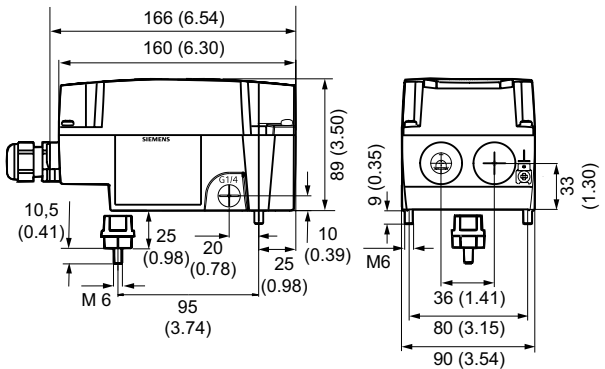
角行程执行机构，尺寸单位：mm
